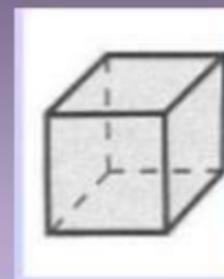
гексаедр
