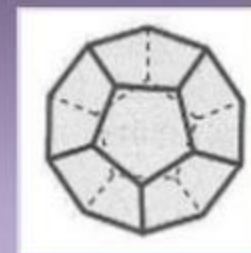
додекаедр
