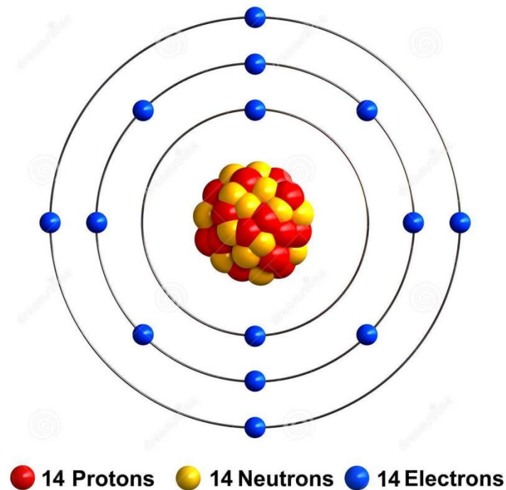
АТОМ КРЕМНИЯ
