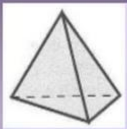
тетраедр
