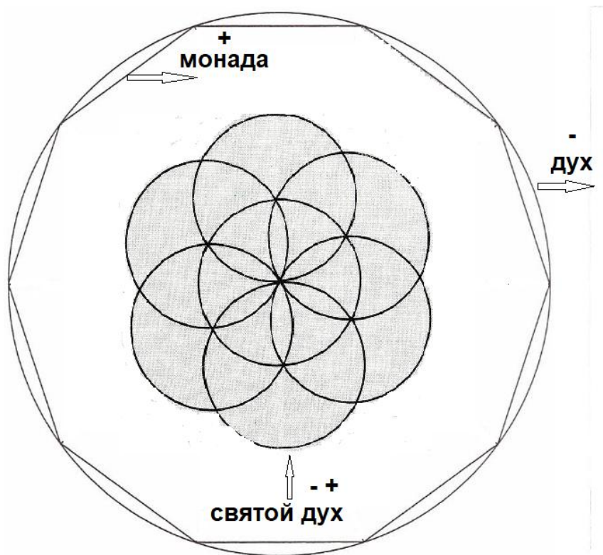
ВСЕЛЕННАЯ
